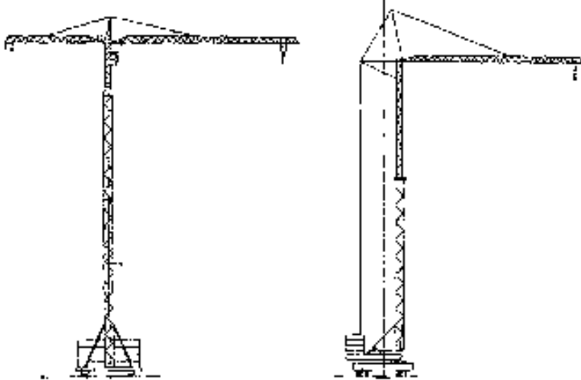
Gru a rotazione in alto
